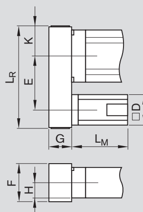
Type RV01, RV02, RV03, RV04
